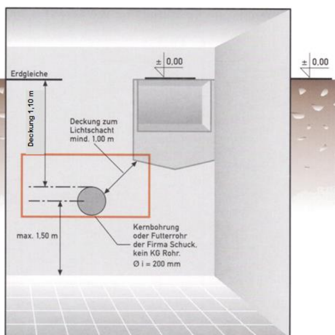
Gebäude mit Keller / Mehrspartenhauseinführung auf freier Wandfläche.
