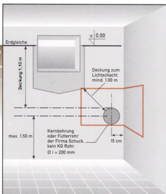
Gebäude mit Keller / Mehrspartenhauseinführung in Raumecke.
